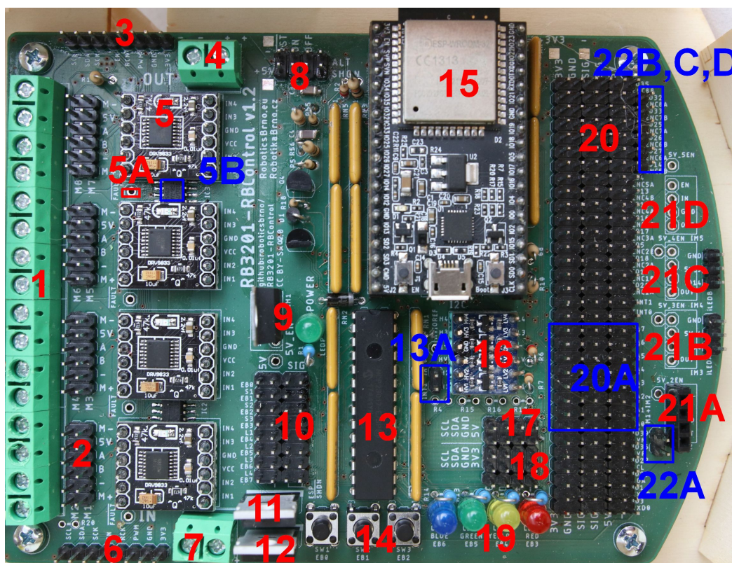
Obrázek 6.1: Rozložení pinů na desce RB3201-RBControl
